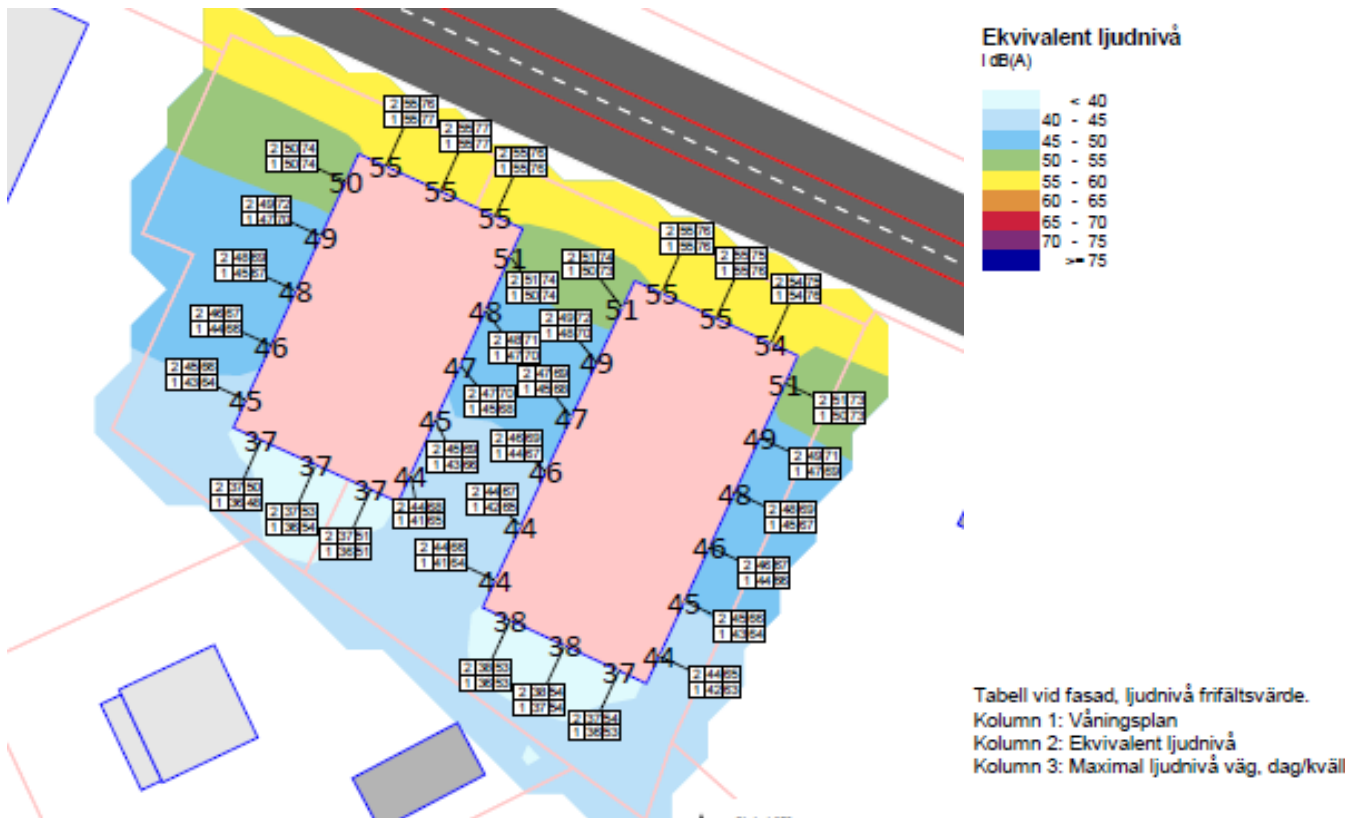
Figur 6. Beräknad ekvivalent ljudnivå vid fasad.
